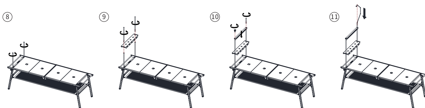
手順は⑧-⑪ラック組立
