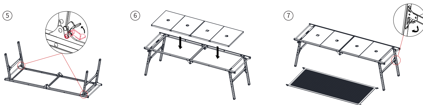
手順⑤-⑦テーブルフレームをロックし、パネルを入れ、物置網を掛ける
