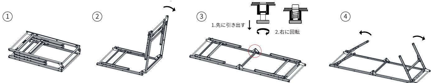
手順①-④オン、ロック
